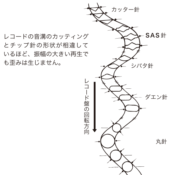
■ 録音再生における各種チップとレコードの音溝の接点
